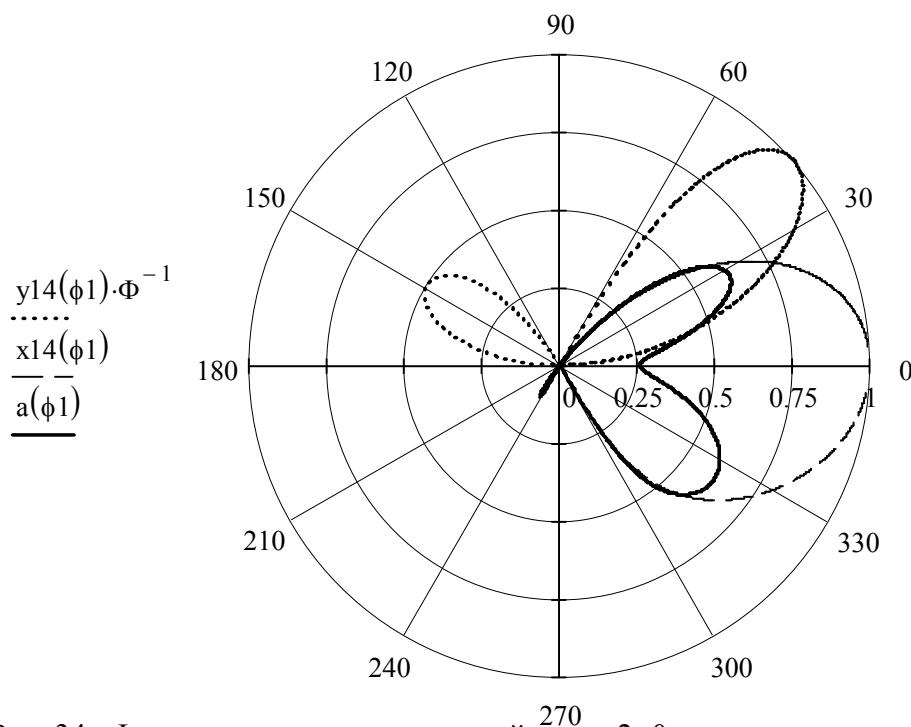
Рис. 34 Функции конечных состояний при m_2=0 в полярных координатах
