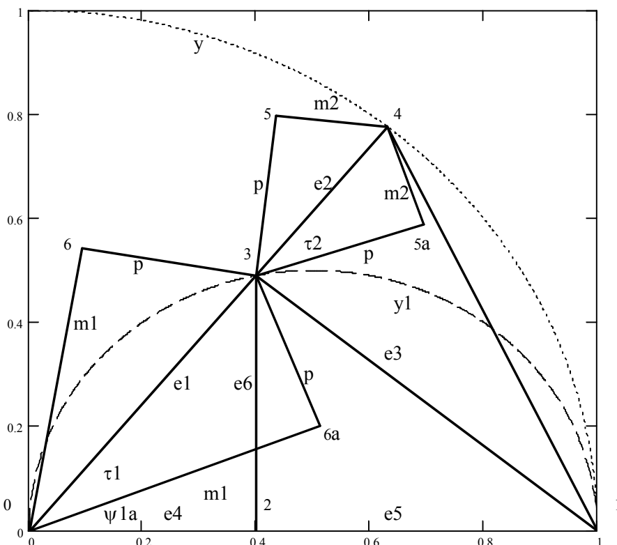
Рис. 35 Схема двухчастичного распада в обе стороны
