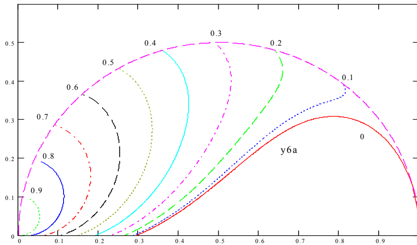
Рис. 38 Семейство кривых y_{ба}(m_1, m_2) от x_{ба}(m_1, m_2) с параметром m_2
